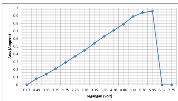
Gambar 20. Hasil pengujian power supply dengan beban 6 ohm.
