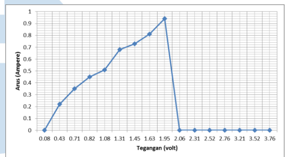
Gambar 16. Hasil pengujian power supply dengan beban 2 ohm.
