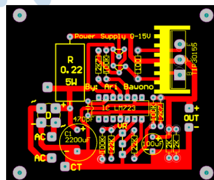
Gambar 6. Desain layout rangkaian regulator tegangan IC LM723
