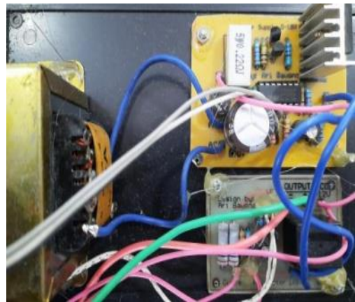
Gambar 10. Pemasangan komponen power supply
