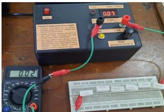
Gambar 14. Konfigurasi pengujian power supply pada beban 6 ohm.
