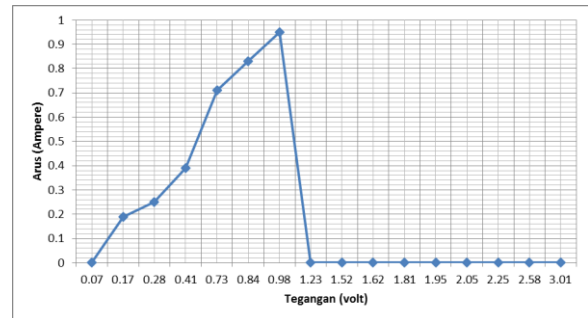
Gambar 15. Hasil pengujian power supply dengan beban 1 ohm.
