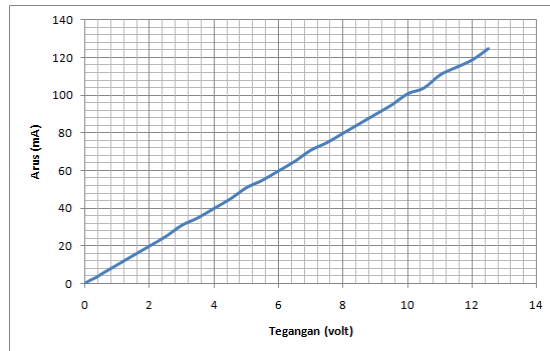
Gambar 13. Hasil pengujian power supply dengan R = 1 \text{ Kohm}
