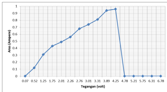
Gambar 18. Hasil pengujian power supply dengan beban 4 ohm.
