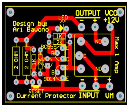
Gambar 7. Desain layout rangkaian proteksi arus lebih DC
