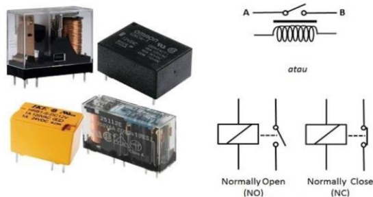
Gambar 4. Bentuk dan simbol komponen relay.
