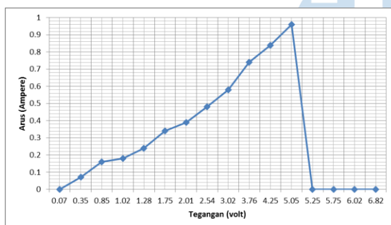
Gambar 19. Hasil pengujian power supply dengan beban 5 ohm.
