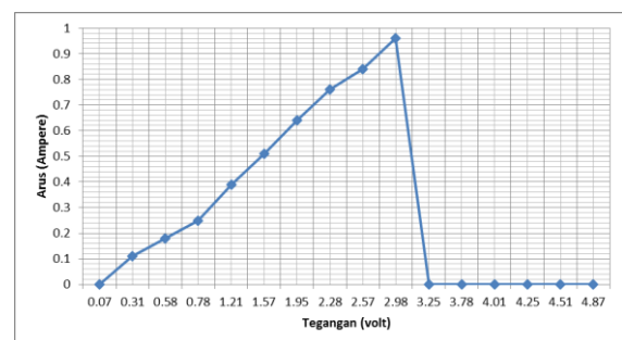
Gambar 17. Hasil pengujian power supply dengan beban 3 ohm.
