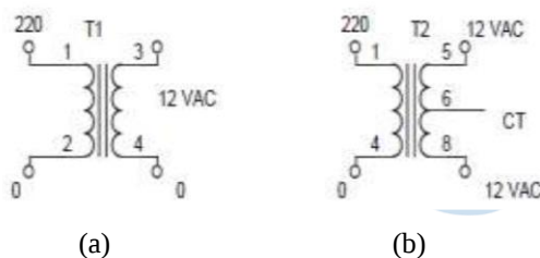
Gambar 1.a). Simbol transformator inti besi tanpa CT b). Transformator inti besi dengan CT
